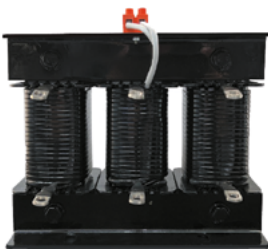
Антирезонансные дроссели
