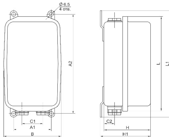
Рисунок 4. Пускатель серии ПМА, IP54
