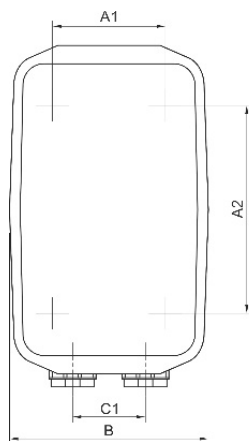
Рисунок 3. Пускатель серии ПМА, IP40
