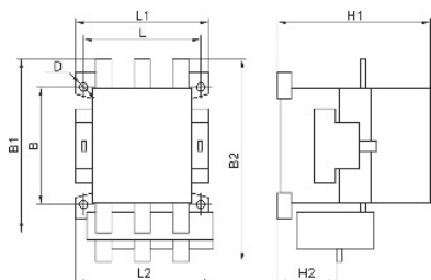
Рисунок 1. Пускатель серии ПМА не реверсивный, IP00
