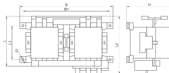
Рисунок 2. Пускатель серии ПМА реверсивный, IP00
